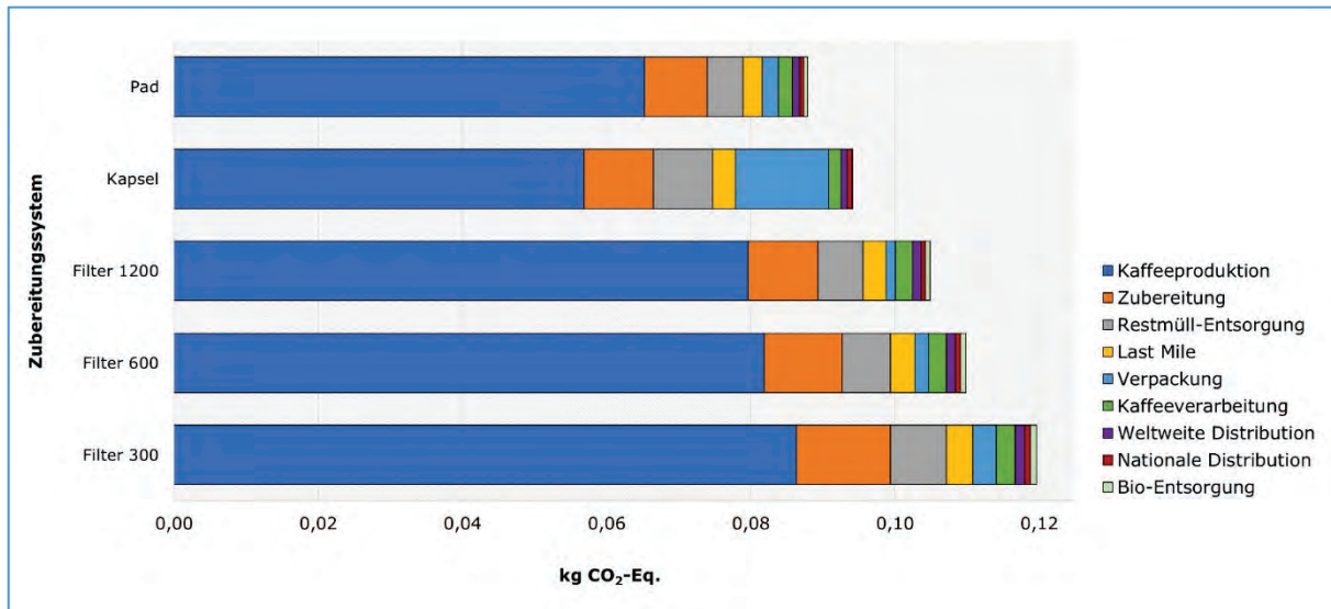
Abb. 2: Umweltauswirkungen in der Wirkungskategorie GWP100 (Klimawandel). Absolute Verteilung der CO 2 -Eq.-Emissionen der verschiedenen Zubereitungssysteme in den einzelnen Lebensweg-Phasen.
