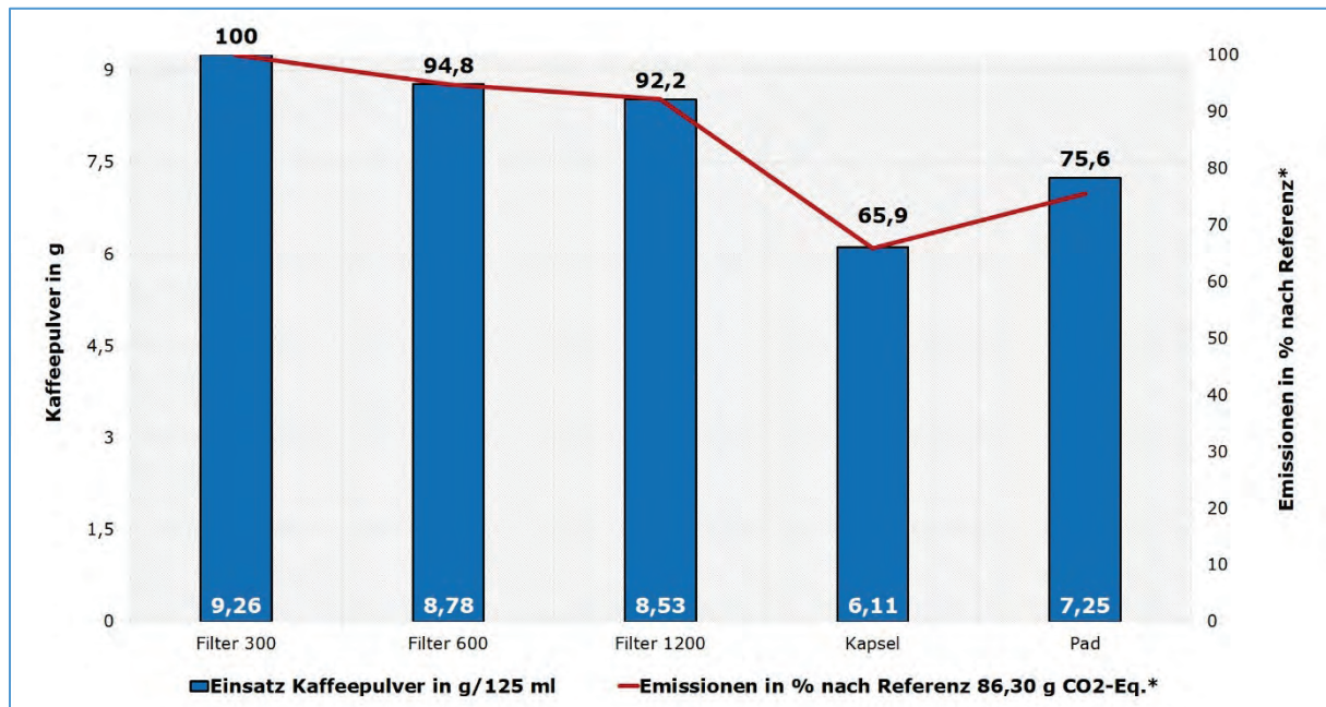
Abb. 4: Eingesetzte Kaffeepulvermengen je 125 ml trinkfertigen Kaffee sowie die damit verbundenen Emissionsschwankungen in % nach Referenz. *Der Höchstwert von 100 % ( \cong 86,30 g erzeugten CO 2 -Eq. beim Filtersystem 300) bildet die Referenz für die anderen Systeme (Bench).
