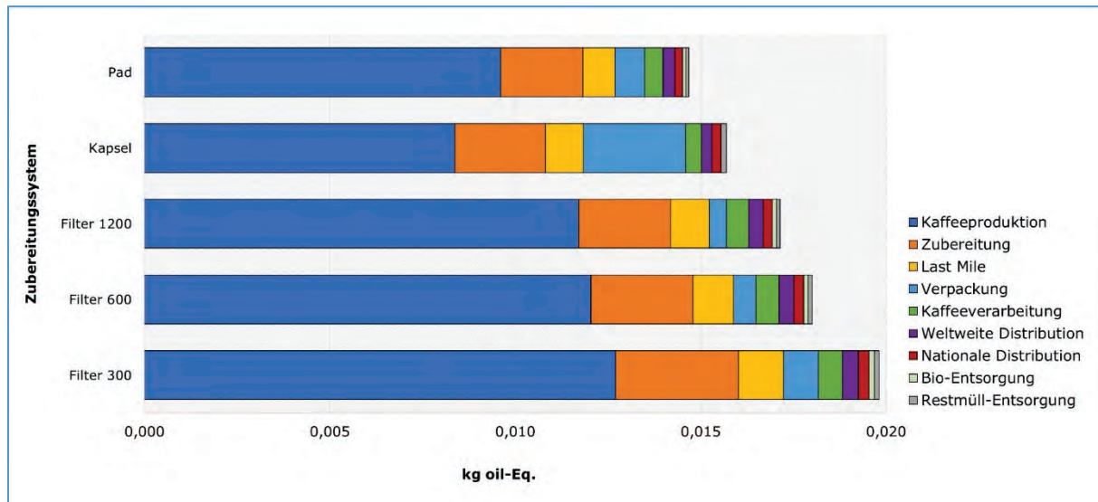
Abb. 5: Umweltauswirkungen in der Wirkungskategorie FDP (Verbrauch fossiler Rohstoffe). Absolute Verteilung der oil-Eq. der verschiedenen Zubereitungssysteme in den einzelnen Lebensweg-Phasen.
